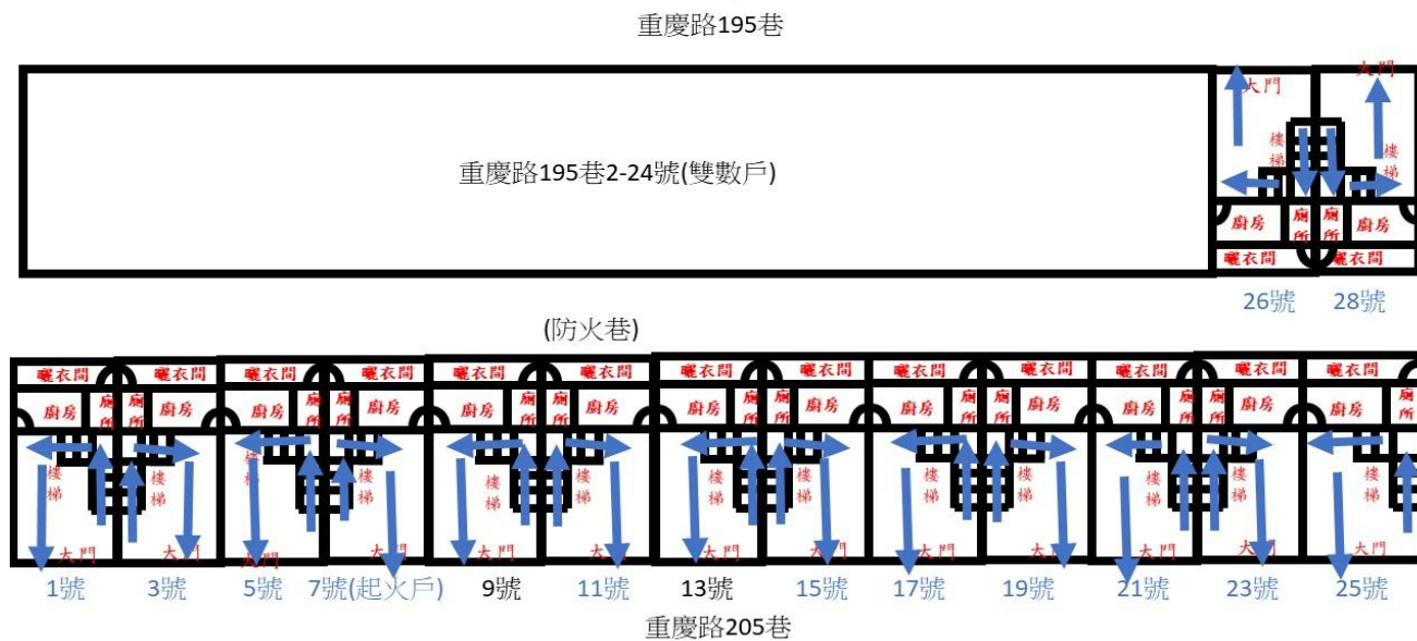
重慶路195及205巷火災案受災戶之1樓平面圖 (藍色字標記為住警器作動之住戶)
