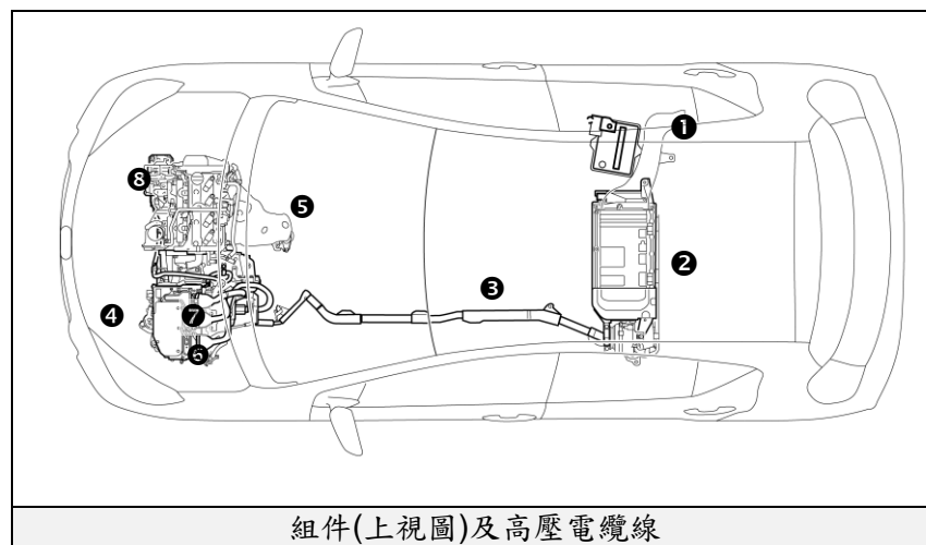
油電複合動力聯合驅動的組件
