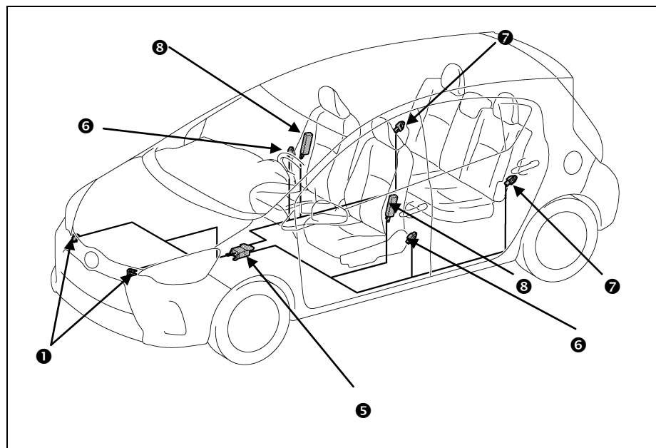
電子式撞擊感知器和側氣囊
